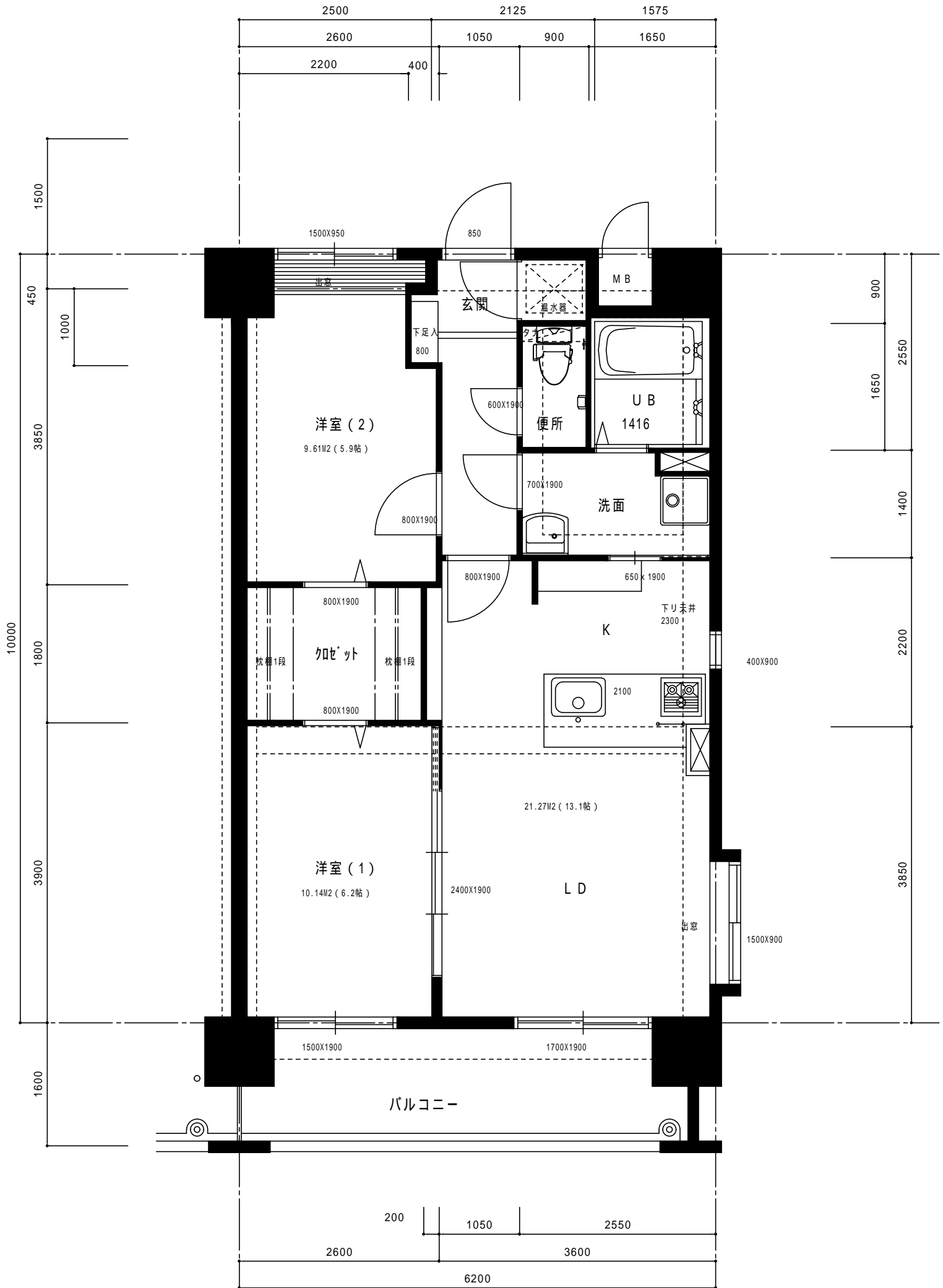
Bタイプ 平面詳細図 (62.00 M 2 )
